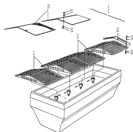
ETB-008071, Ruszty sitowe górne
