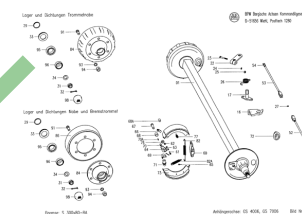
ETB-008090, Oś hamowana, 8 t, hamulec najazd., rozstaw kół 1850, firma BPW
