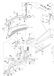
ETB-008088, Rozsiewacz granic, lewy "Limiter ZG-B1"
