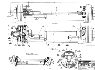
ETB-008090, Oś hamowana, 8 t, hamulec najazd., rozstaw kół 1850, firma BPW
