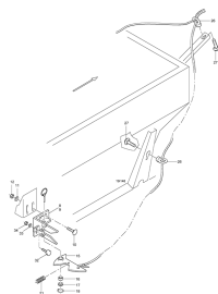
ETB-008044, Przedni ślimak rozsiewający FS 9 m (7/7)
