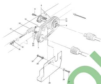
ETB-008008, Napęd pośredni
