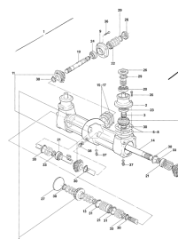
ETB-008025, Uniwersalna przekładnia rozsiewająca (1/2)
