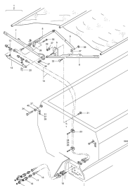
ETB-008068, Składana plandeka, obsługa hydr. 6001-10001
