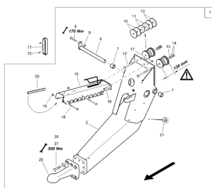
ETB-007995, Dyszel z zaczepem kulowym
