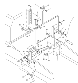
ETB-008001, Regulacja zasuwn, od
