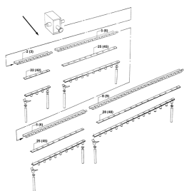
ETB-008055, Przedni ślimak rozsiewający FS 12 m (11/17)
