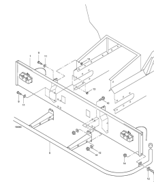
ETB-008018, Ściana tylna / pałąk ochronny
