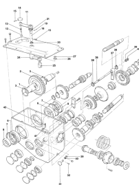
ETB-008023, Skrzynia biegów do regulacji prędkości taśmy
