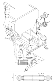
ETB-008065, Napęd od koła jezdnego (2/2)
