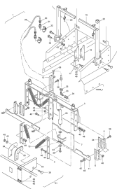
ETB-008003, Podwójne zasuwy, hydr. - jednostr. Wyłączanie, od 01/2001
