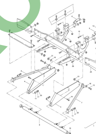
ETB-008081, Zabezpieczenie przeciwwjazdowe do ZG-B 20001 T
