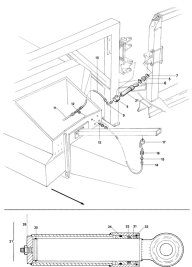
ETB-008051, Przedni ślimak rozsiewający FS 12 m (7/17)
