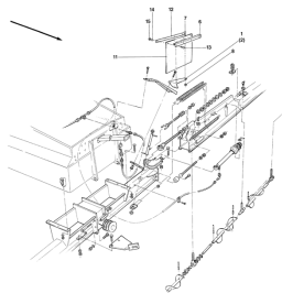
ETB-008039, Przedni ślimak rozsiewający FS 9 m (2/7)
