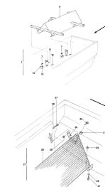
ETB-008070, 1. zadaszenie odciażające taśmę 2. ruszty sitowe dolne
