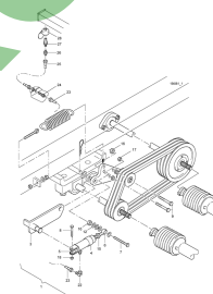
ETB-008009, Sprzęgło odłączające Hydro
