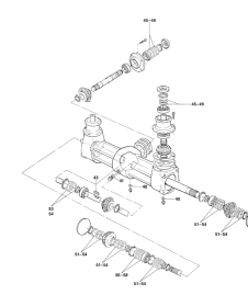
ETB-008026, Uniwersalna przekładnia rozsiewająca (2/2)
