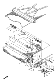
ETB-008015, Taśma, od 1998, (2/2)
