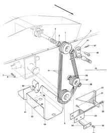
ETB-008063, Przedni ślimak rozsiewający FS 9 m i FS 12 m
