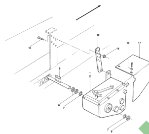
ETB-008020, Skrzynia biegów do regulacji prędkości taśmy przenośnika, elementy montażowe
