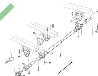
ETB-008006, Wałek napędu głównego (2/2)
