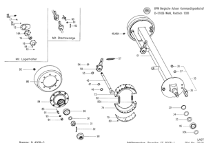
ETB-008091, Oś hamowana, 8 t, 25 km/h, rozstaw kół 1850, firma BPW
