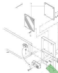
ETB-008077, Tablica ostrzegawcza do nadwymiarowej szerokości
