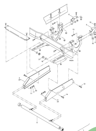
ETB-008080, Zabezpieczenie przeciwwjazdowe, od 04.1998
