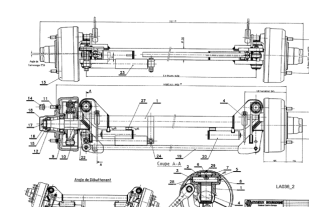
ETB-008093, Oś tandemowa hamowana 25 km/h, 16 t, rozstaw kół 1900, 1/3
