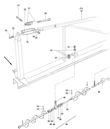
ETB-008052, Przedni ślimak rozsiewający FS 12 m (8/17)
