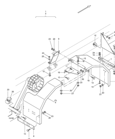
ETB-008085, Błotniki 700 ZG-B1
