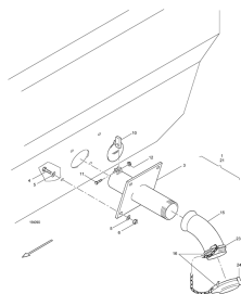
ETB-008076, Króciec wdmuchujący
