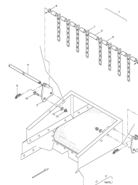
ETB-008073, Grabie łańcuchowe do nawozu ZG-B1
