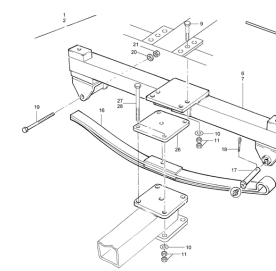
ETB-007998, Zawieszenie do osi ZG-B 8000/10000 kg
