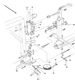
ETB-008049, Przedni ślimak rozsiewający FS 12 m (5/17)
