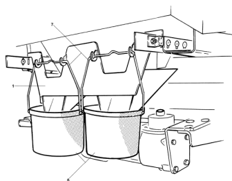
ETB-008075, Urządzenie do ustawiania odpowiedniej dawki rozsiewu
