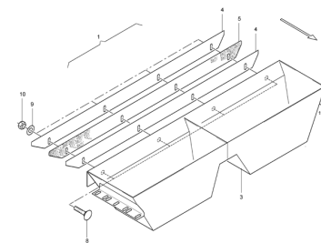
ETB-008062, Przedni ślimak rozsiewający FS 9 m i FS 12 m
