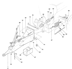
ETB-007991, Dyszel najazdowy AVE-2000 z automatyką cofania
