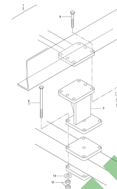
ETB-008089, Kocioł mocowania osi, 280 mm
