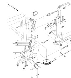
ETB-008050, Przedni ślimak rozsiewający FS 12 m (6/17)
