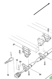
ETB-008005, Wałek napędu głównego (1/2)
