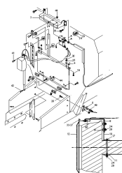
ETB-008004, Regulacja zasuw, elektr. (regulacja dawki) od 01/2001
