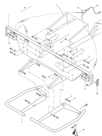
ETB-008019, Ściana tylna, od 03.2001 / oświetlenie
