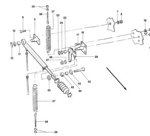
ETB-008058, Przedni ślimak rozsiewający FS 12 m (14/17)
