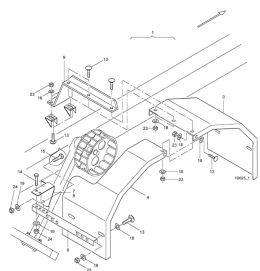
ETB-008083, Błotniki - napęd od koła jezdnego, pojedynczy
