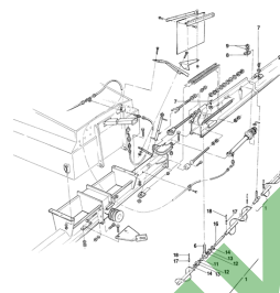
ETB-008041, Przedni ślimak rozsiewający FS 9 m (4/7)
