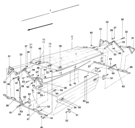
ETB-008067, Składana plandeka, obsługa mech. 12001/16001
