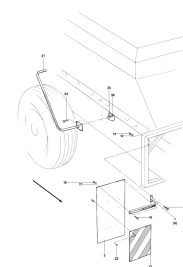
ETB-008061, Przedni ślimak rozsiewający FS 12 m (17/17)
