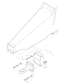
ETB-008078, Wspornik do przesuwania dysza pociągowego
