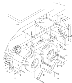
ETB-008087, Błotniki 700 ZG-B 20001
