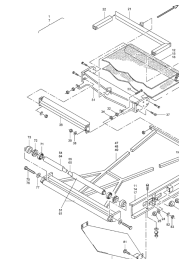
ETB-008014, Taśma, od 1998, (1/2)
