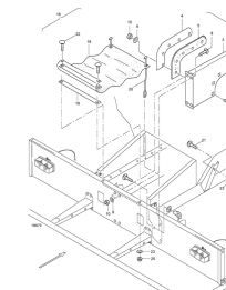
ETB-008074, Rozdzielacz strumienia nawozu / plandeka ZG-B1
