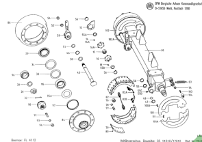
ETB-008092, Oś hamowana, 10 t, 25/40 km/h, rozstaw kół 1850, firma BPW
