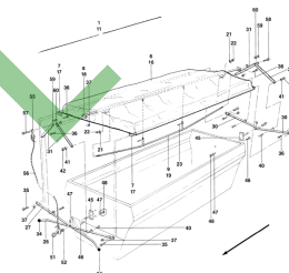
ETB-008066, Składana plandeka, obsługa mech. 6001-10001
