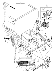
ETB-008064, Napęd od koła jezdnego (1/2)
