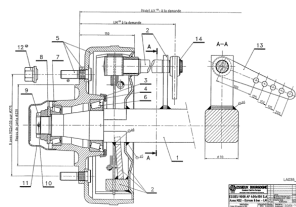
ETB-008095, Oś tandemowa hamowana 25 km/h, 16 t, rozstaw
