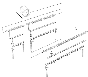
ETB-008043, Przedni ślimak rozsiewający FS 9 m (6/7)
