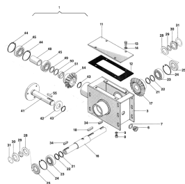
ETB-008047, Przedni ślimak rozsiewający FS 12 m (3/17)
