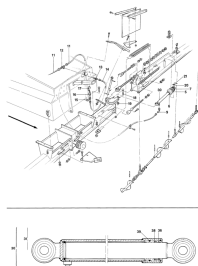
ETB-008040, Przedni ślimak rozsiewający FS 9 m (3/7)
