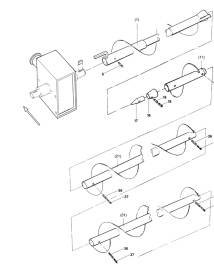
ETB-008042, Przedni ślimak rozsiewający FS 9 m (5/7)
