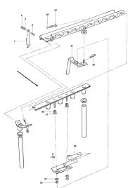
ETB-008056, Przedni ślimak rozsiewający FS 12 m (12/17)
