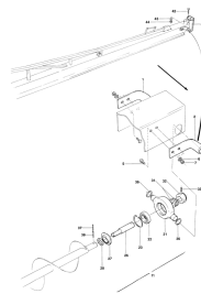
ETB-008053, Przedni ślimak rozsiewający FS 12 m (9/17)
