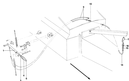
ETB-008059, Przedni ślimak rozsiewający FS 12 m (15/17)
