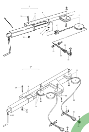
ETB-007996, Hamulec postojowy do ZGB z hamulcem pneum./ham. post. II
