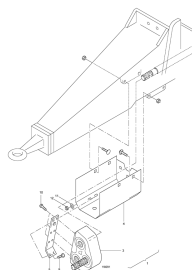
ETB-008007, Napęd od WOM-u 1000 obr./min
