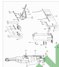
ETB-007993, Dyszel najazdowy
