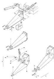
ETB-007992, Dyszel pociągowy prosty, 150 mm, wysoki dyszel Hitch - dyszel z zaczepem kulowym
